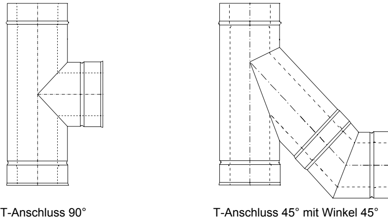
Bild 8: Anschluss an senkrechter Abgasanlage
