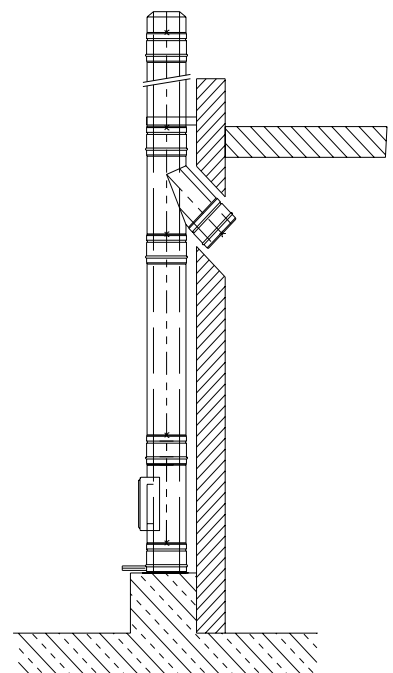
Bild 7: Aufbau mit Grundplatte für Sockelmontage
