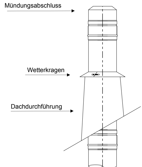
Bild 11: Dachdurchführung
